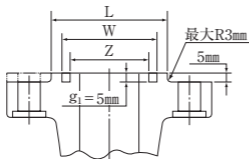
ラージ グループ座
