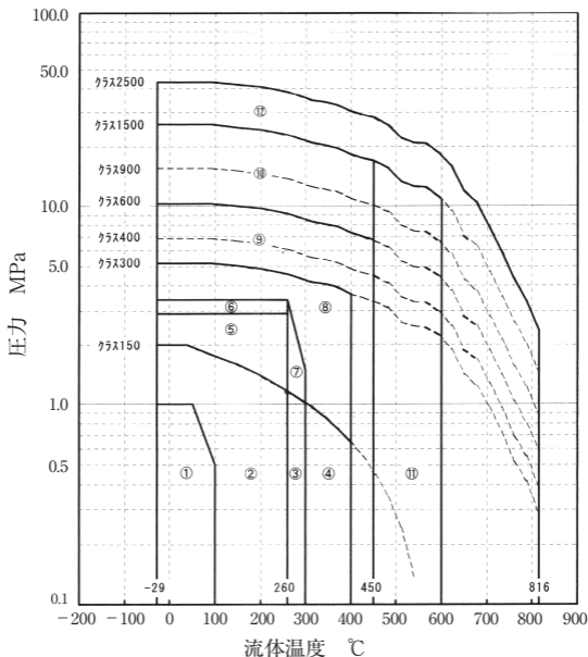
図4 ガスケット選定図 (ガス系流体 I)
