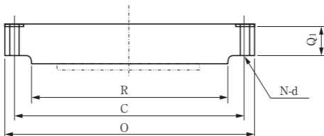
ブラインド形フランジ
