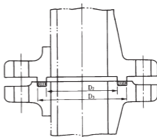
溝形フランジ用
