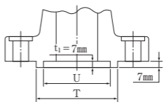
スモール グループ座
