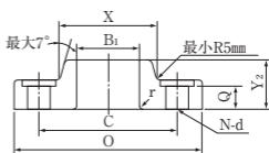
ソケット溶接形
