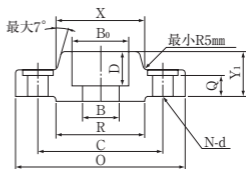
ソケット溶接形
