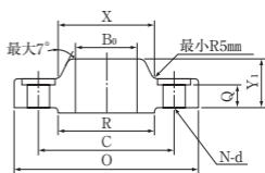
スリップオン形
