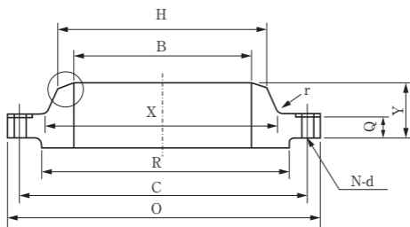
突合せ溶接形フランジ
