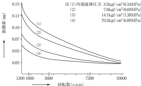
回転軸における振動量と回転数の関係
