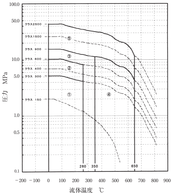
図11 グランドパッキン選定図（ガス系流体 I、II） (1)
