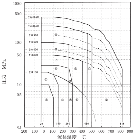
図2 ガスケット選定図（油系流体）
