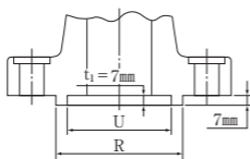
ラージ グループ座
