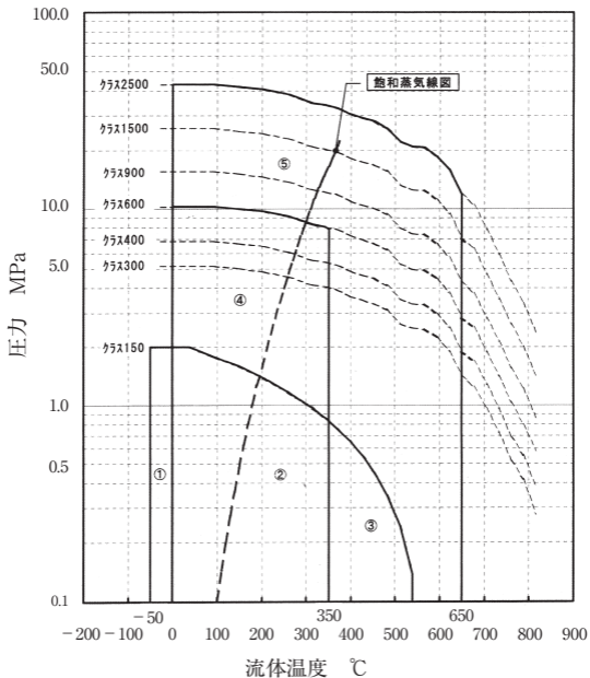
図7 ガスケット選定図（水系流体・油系流体・腐食性流体・ガス系流体 I、II）
