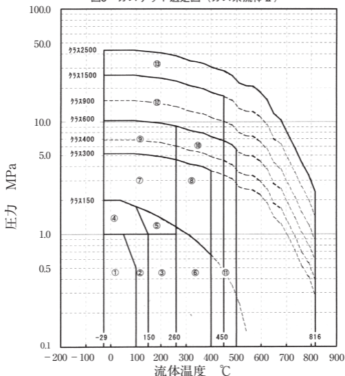
図5 ガasket選定図（ガス系流体Ⅱ） (1)
