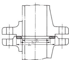
はめ込み形フランジ用
