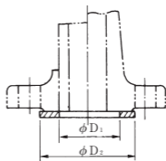
大平面座フランジ用
