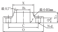
ソケット溶接形
